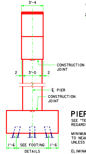
END ELEVATION
