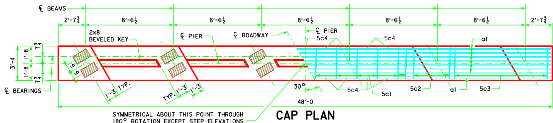
CAP PLAN
