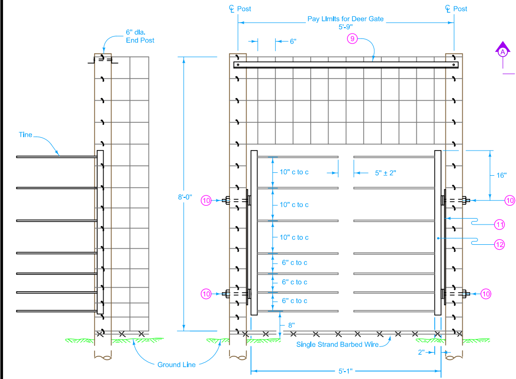
SECTION A-A
