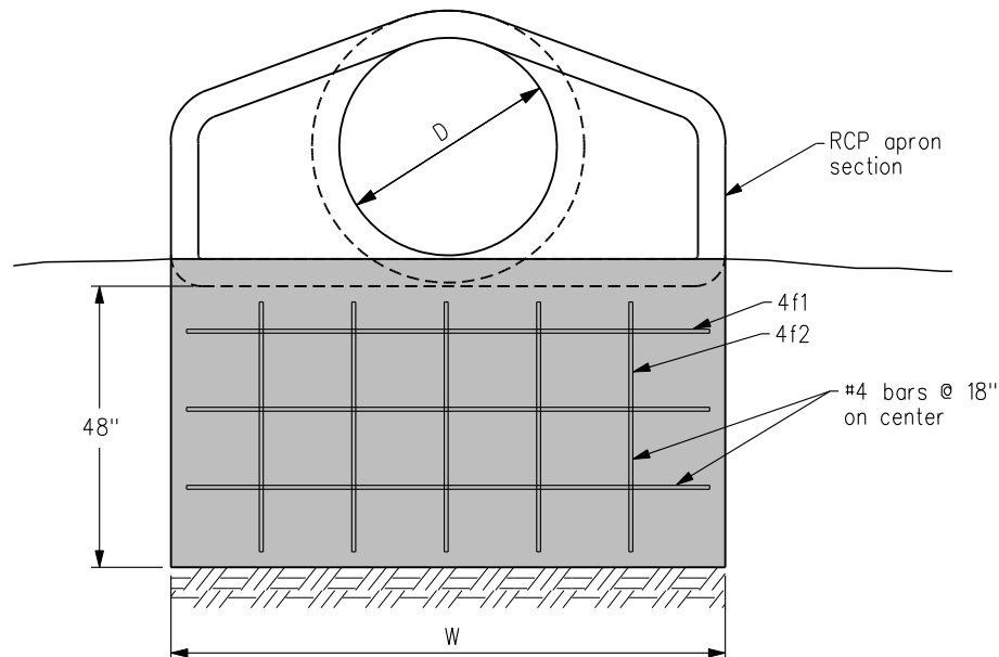
ELEVATION
