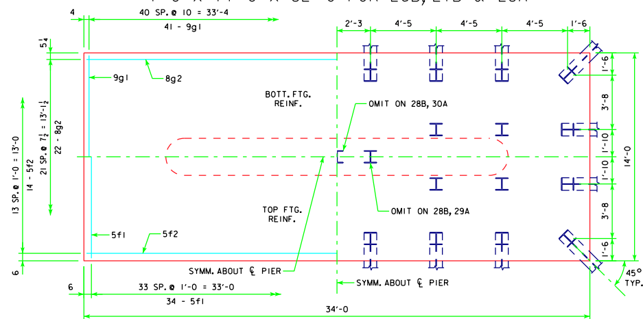
4'-0 x 14'-0 x 34'-0 FOR 28B, 29A & 30A
