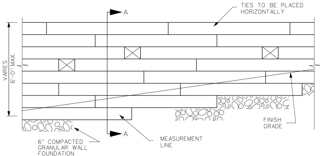
ELEVATION
