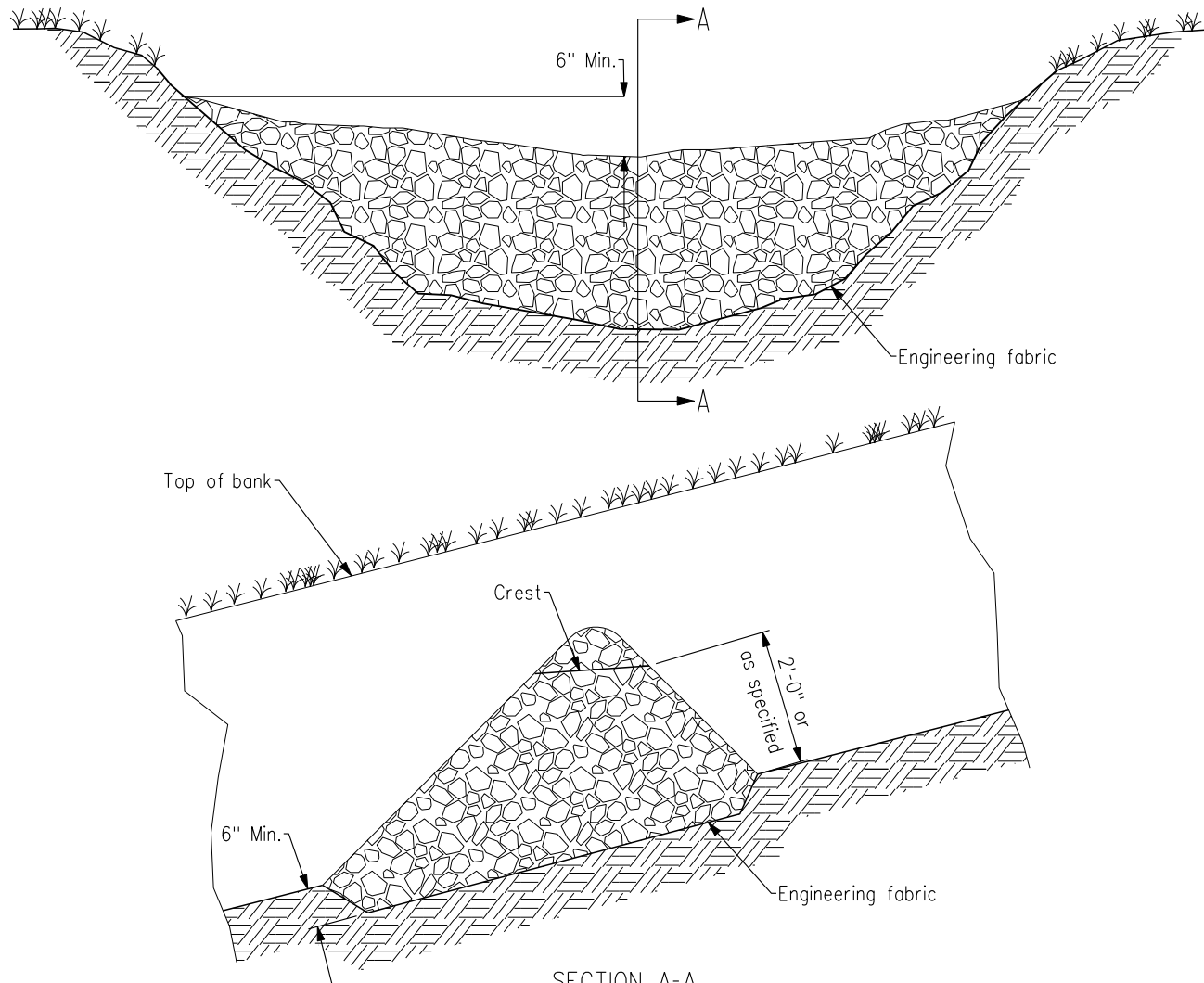
SECTION A-A
