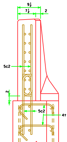
VIEW A-A
